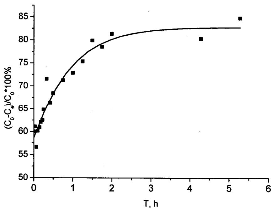
Fig. 2. Gradul de purificare a apelor de ioni de nitriți în funcție de timpul de aerare
