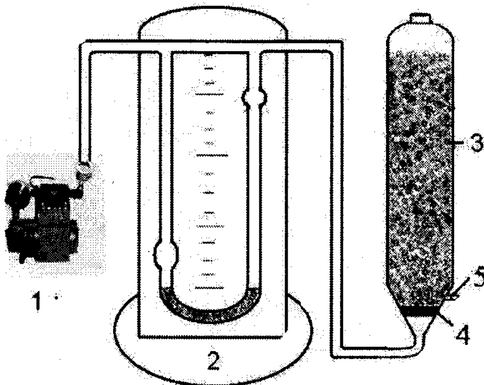
Fig. 1. Schema instalației pentru aerarea apelor de nitriți cu pat fluidizant de catalizator
